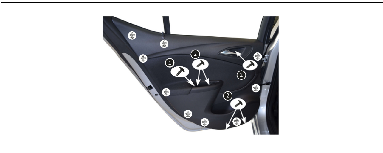
Bild 1: Übersicht Türverkleidung hinten
